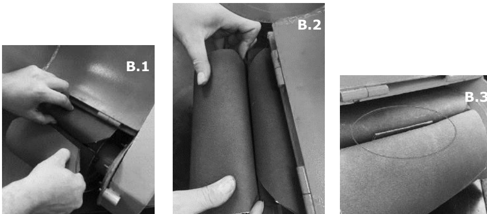
B) Schleifband um die Rolle wickeln (B.1) und die Enden in die Öffnungen stecken (B.2). Bei normalem Schleifpapier muss der entstandene Spalt ausgefüllt werden (B.3). Dies macht man am besten mit einem Stück gefalteten Papier. Bei stärkeren Schleifmitteln (z.B. Schleif-Fließ) Platzhalter weggelassen.
